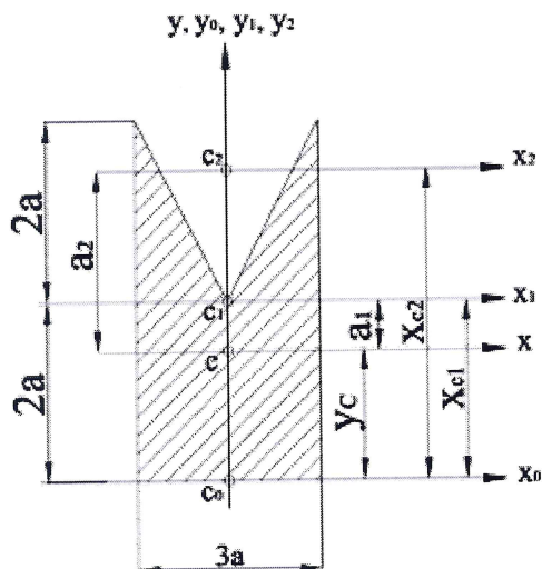
Рис. 1 – Схема поперечного сечения
